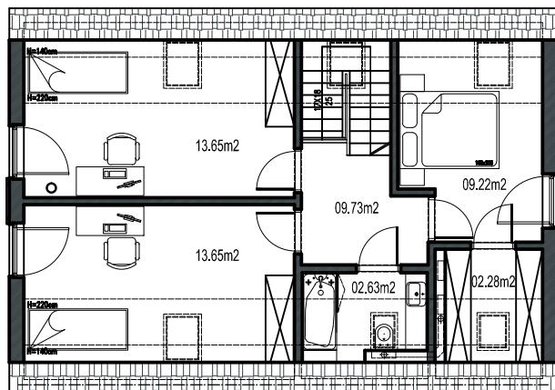
RZUT PODDASZA
