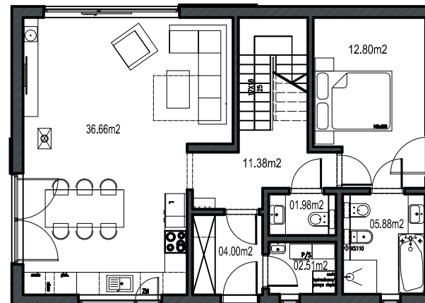
RZUT PARTERU
