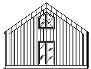
ELEWACJA SZCZYTOWA
