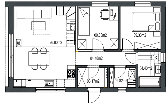
RZUT PARTERU
