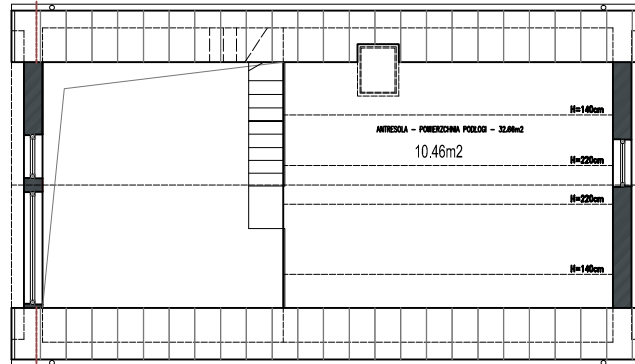
RZUT ANTRESOLI
