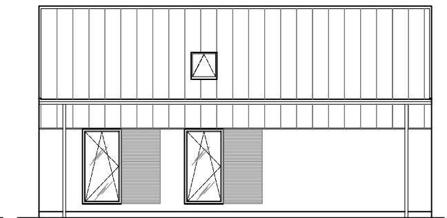
ELEWACJA BOCZNA
