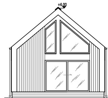
ELEWACJA SZCZYTOWA
