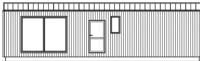
ELEWACJA FRONTOWA
