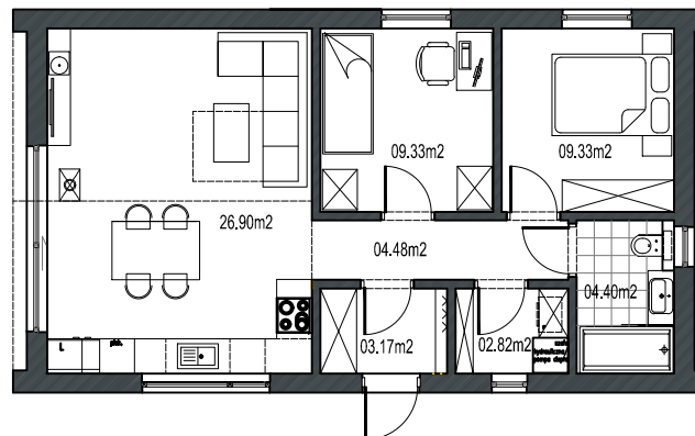
RZUT PARTERU
