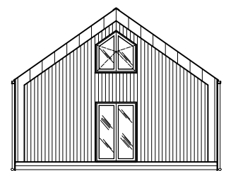
ELEWACJA SZCZYTOWA
