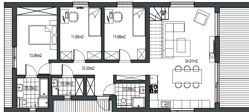
RZUT PARTERU
