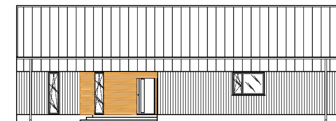
ELEWACJA FRONTOWA
