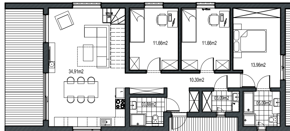
RZUT PARTERU
