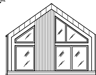
ELEWACJA SZCZYTOWA
