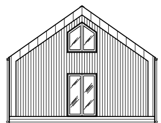
ELEWACJA SZCZYTOWA
