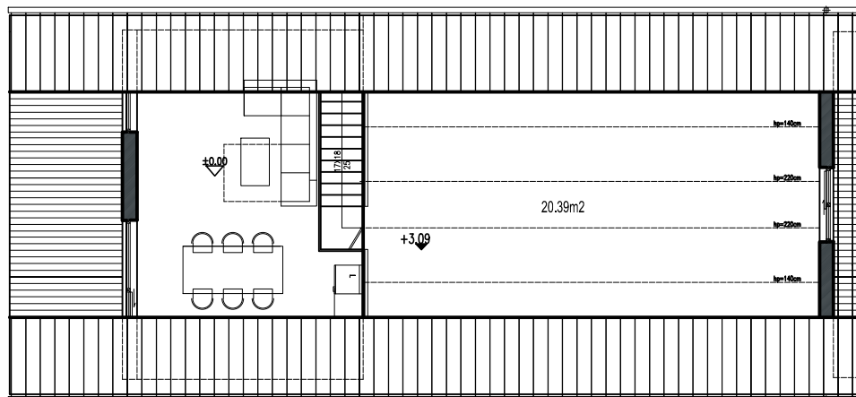
RZUT ANTRESOLI
